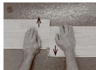
Afmontering Top Connect: Elementerne kan skubbes parallelt fra hinanden.
